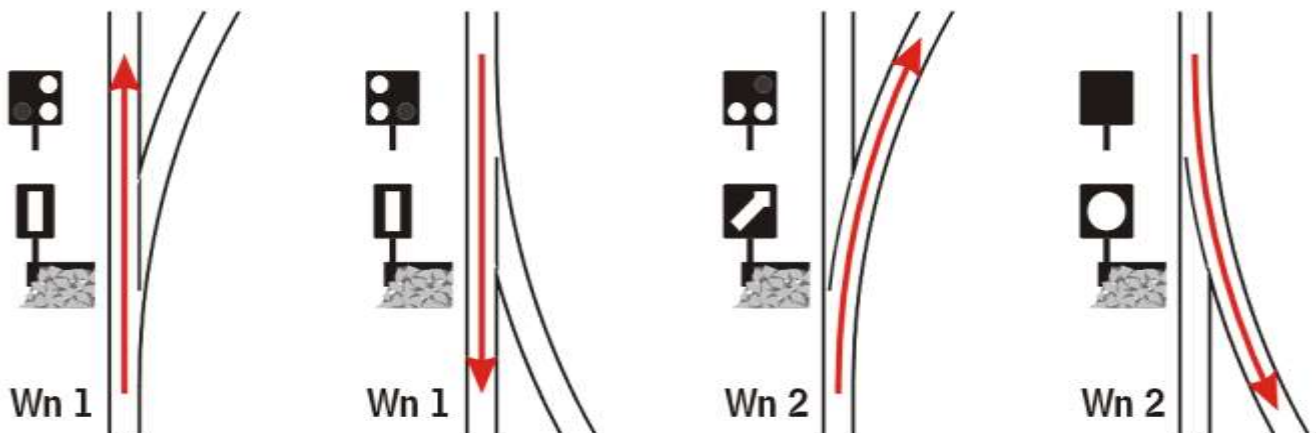
Figure 1: Quelle: https://de.wikipedia.org/wiki/Weichensignal
